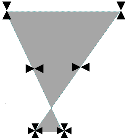
Kuva 7. Tähykslinjojen geometria. Kun kameran projektiokeskus on tähykslinjojen leikkauspisteessä ja niiden muodostamassa tasossa (harmaa), tähykset muodostavat kuvalle ristin muotoiset kuviot.
